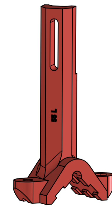
AllgSicht2 Maßstab 1:5
