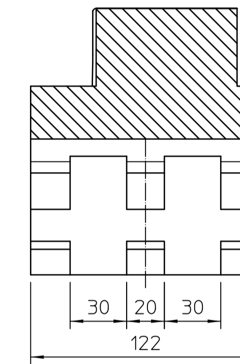
Schnitt B-B
