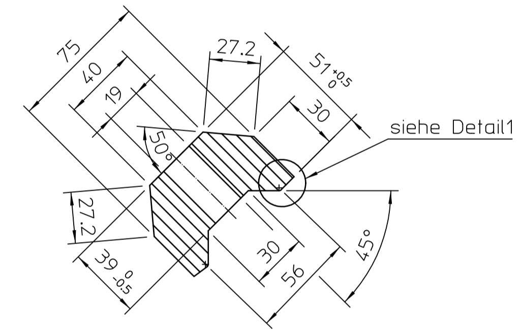
Schnitt D-D
