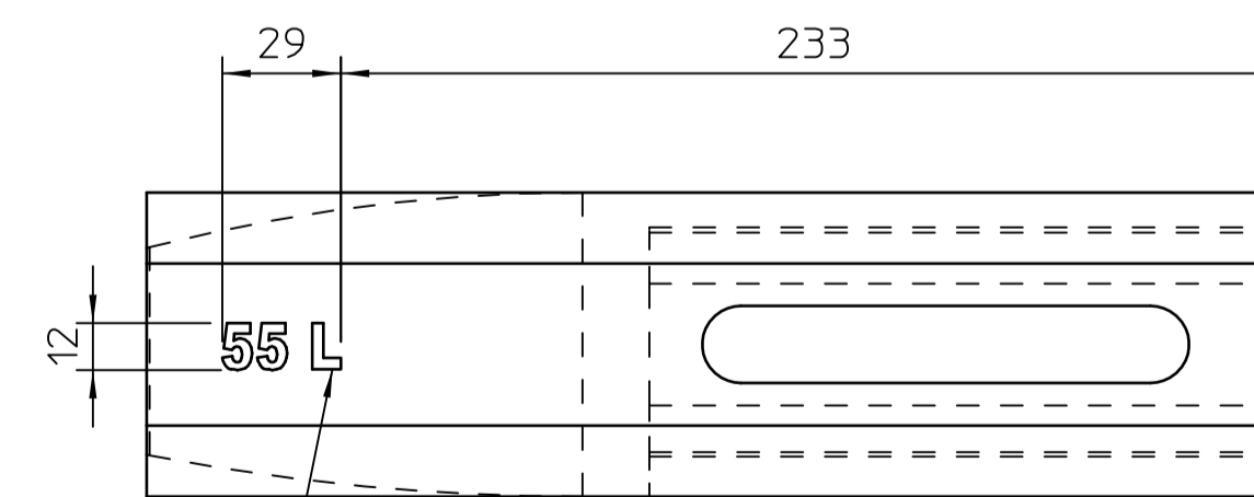
Teilansicht1 Maßstab 1:2 1,5 tief 1,5 深
