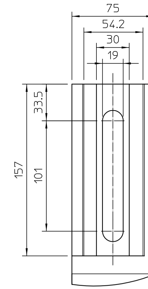
Teilansicht1 Maßstab 1:2
