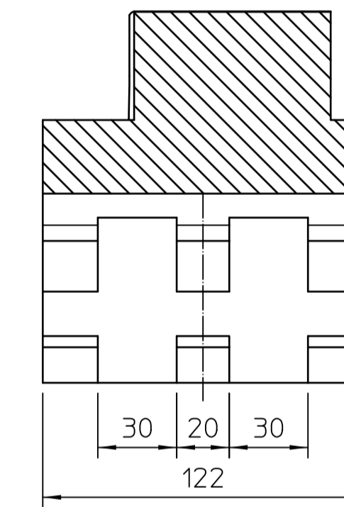
Schnitt B-B
