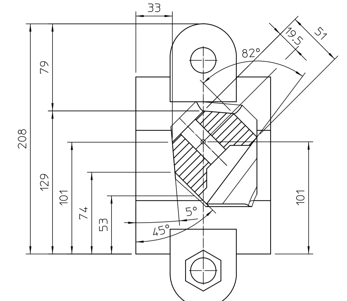
Schnitt C-C
