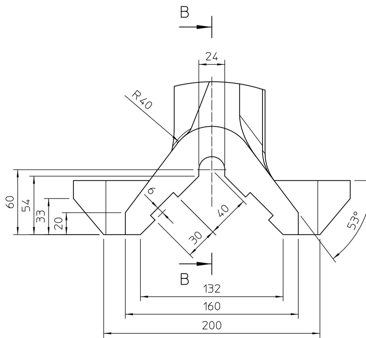
Teilansicht2 Maßstab 1:2
