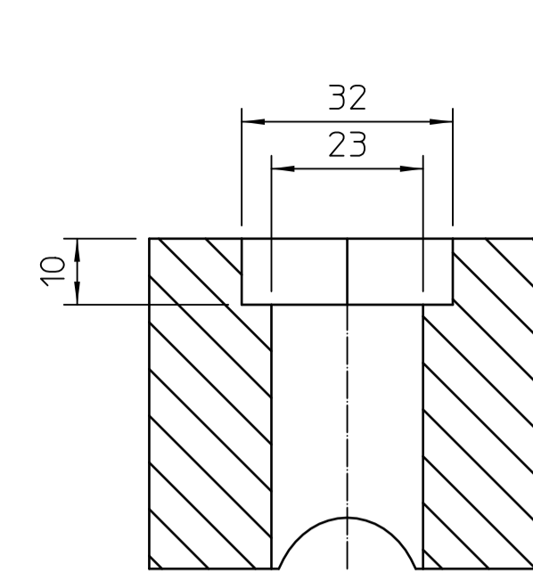
Schnitt A-A Maßstab 1:1
