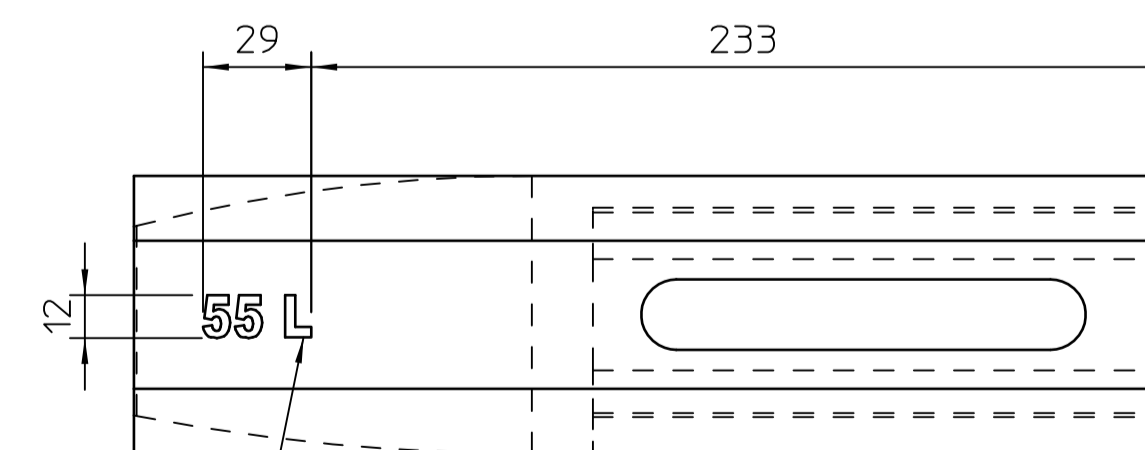
1,5 tief 1,5 深 Teilansicht1 Maßstab 1:2
