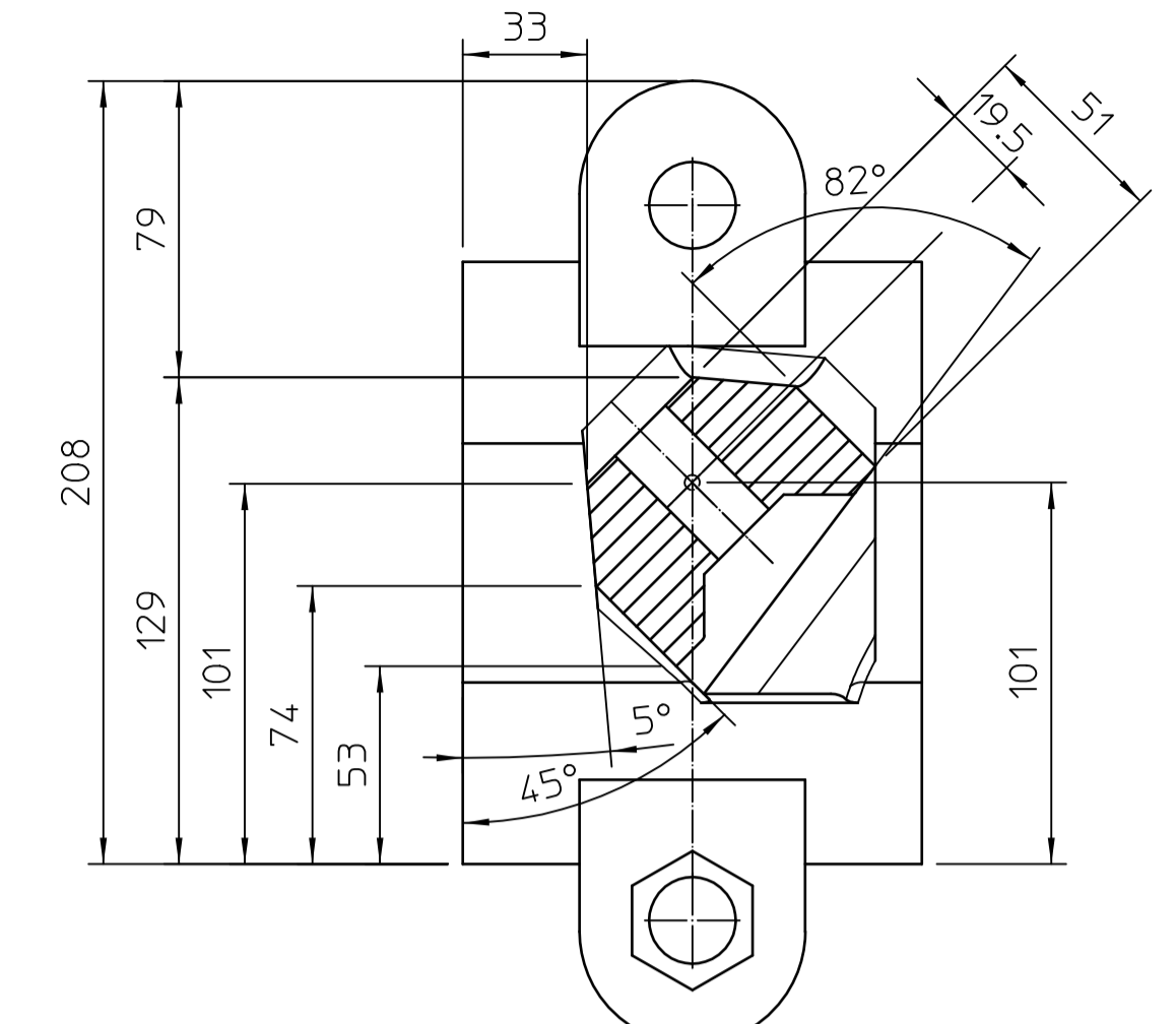
Schnitt C-C
